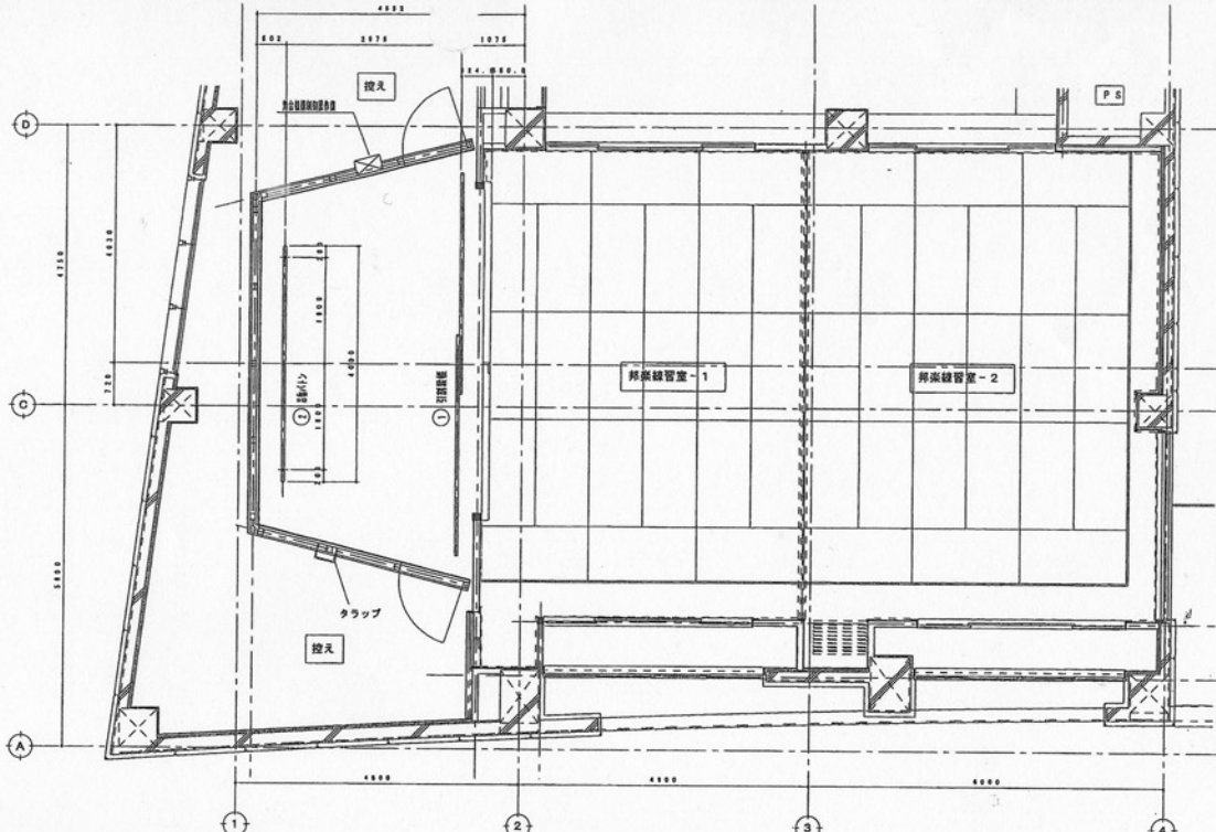
平面配置図
