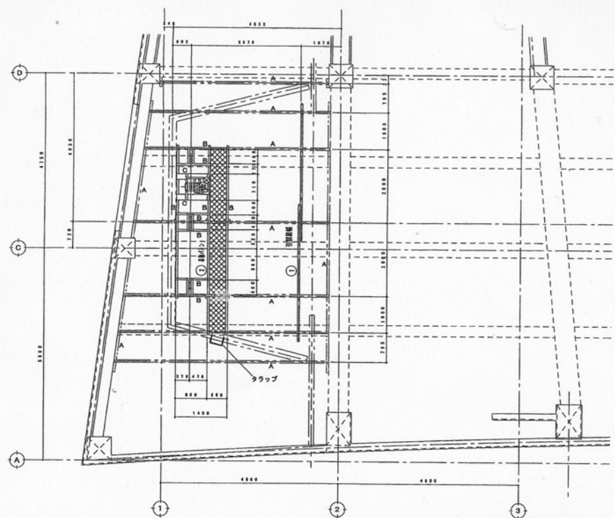
すのこ機器配置図
