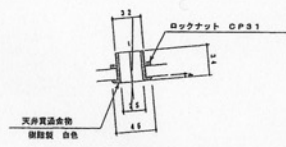
天井貫通金物詳細
