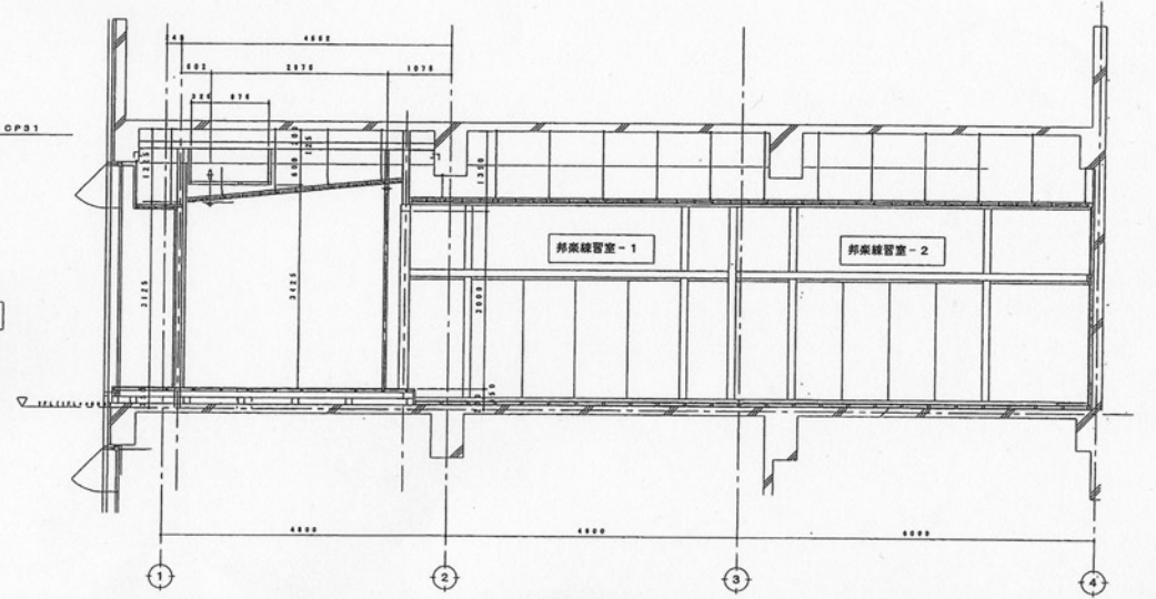
断面配置図
