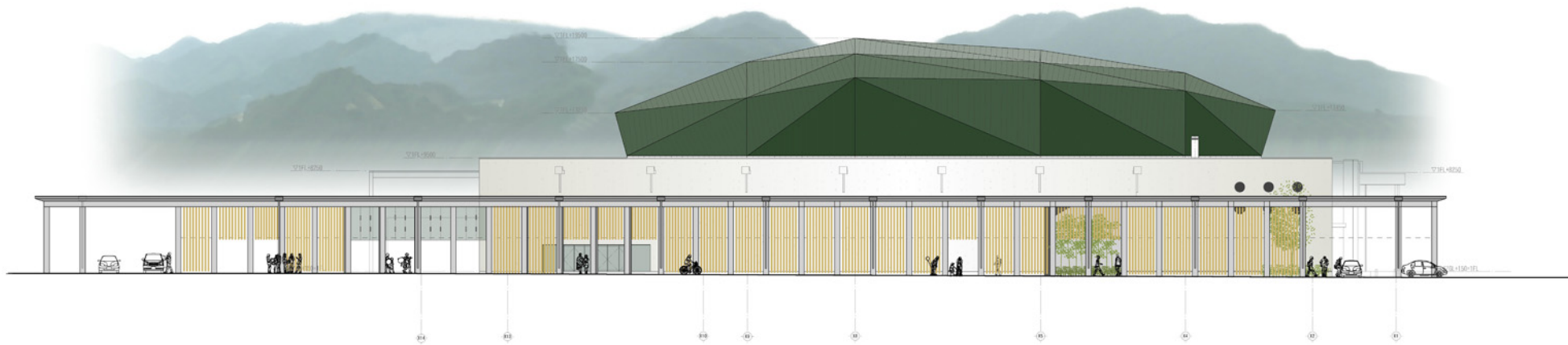
北側立面圖 A2=1/200 (広場側)
